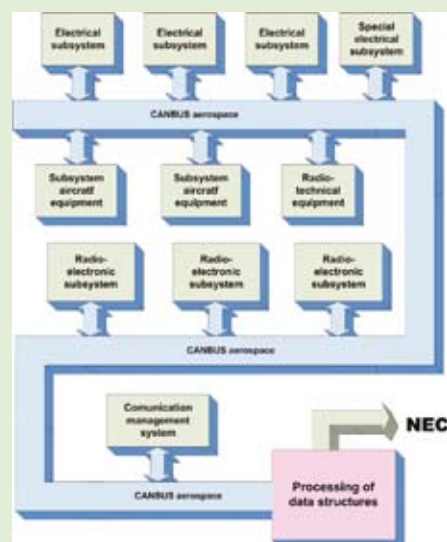
Obr. č. 1 Ideová struktura leteckého palubního elektronického systému
