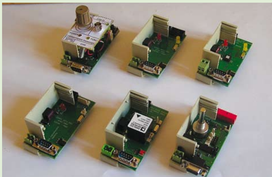
Obr. č. 2 Ukázka sestavy avionických modulů určených pro montáž na DIN
