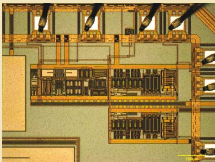
Snímek čipu pořízen laserovým konfokálním mikroskopem OLYMPUS LEXT OLS 3000.
