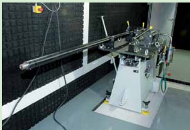
Pneumatický urychlovač projektilů
